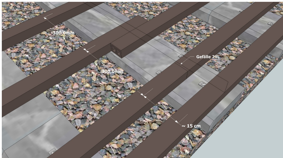
Abb.1: Unterbau und Unterkonstruktion, z.B. Betonsteine und BPC UK-Rahmen
