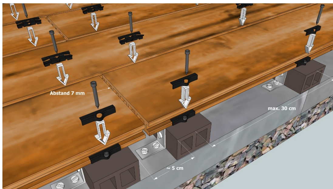
Abb. 2: Befestigung der Dielen auf der Unterkonstruktion
