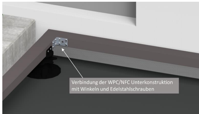
Bild 7. Mit handelsüblichen Winkeln z.B. 35 x 50 x 50 mm kann eine stabile Rahmenkonstruktion erstellt werden.
