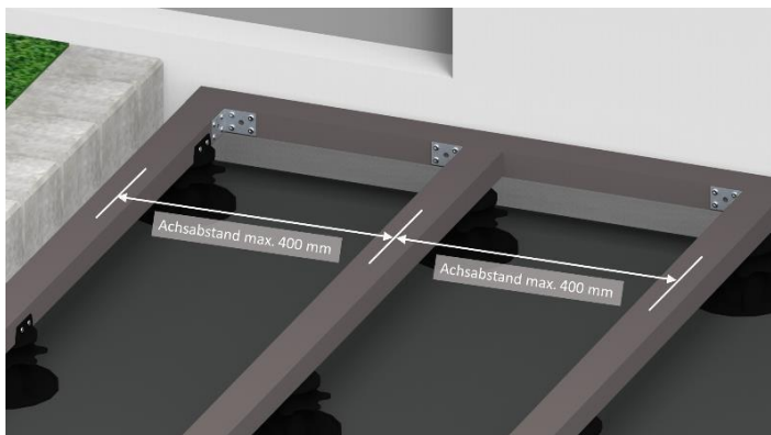
Bild 8. Der Achsabstand der Unterkonstruktionen darf 300 mm nicht überschreiten. ACHTUNG: Bildbezeichnung 400 mm, jedoch gilt 300 mm Achsabstand.
