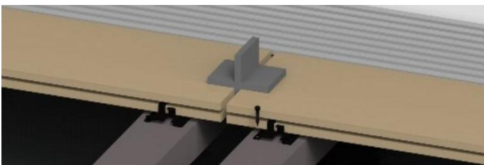
Bild 16. Mit handelsüblichen Abstandhaltern können gleichmäßige Fugenabstände an den Längsstößen der WPC-Dielen sichergestellt werden. Die Abstände sind von der Verlegetemperatur der WPC-Dielen abhängig.
