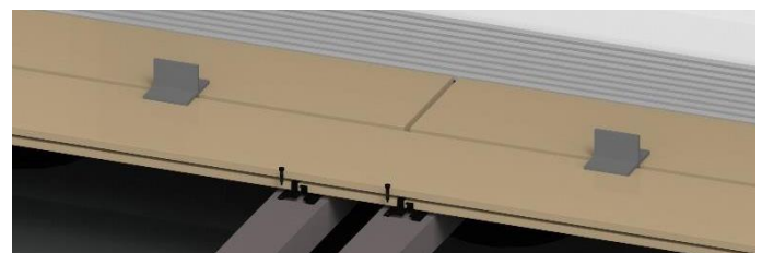
Bild 17. Mit Abstandshaltern kann einfach eine ca. 1 mm größere Fuge sichergestellt werden als die Befestigungssysteme vorgeben.
