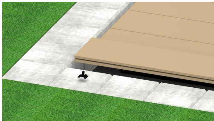
Bild 29. Bevor die letzte WPC-Diele eingesetzt wird, müssen alle Anfangs-/Endclipse auf die WPC-Diele gesteckt werden.
